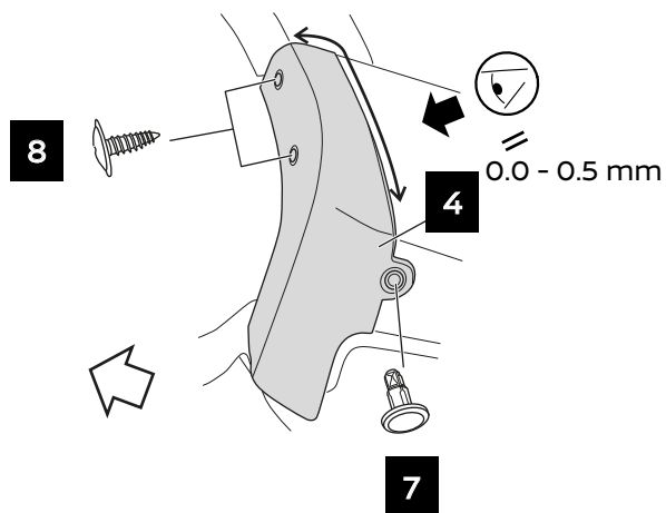
MUDGUARD RR LH & RH (Fig.16 - Fig.17)
