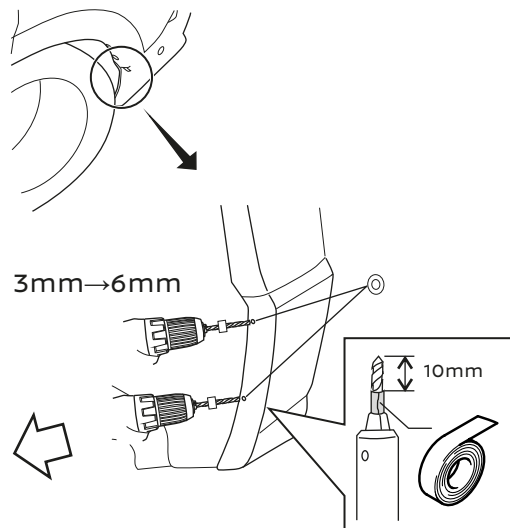
MUDGUARD RR LH & RH (Fig.16 - Fig.17)
